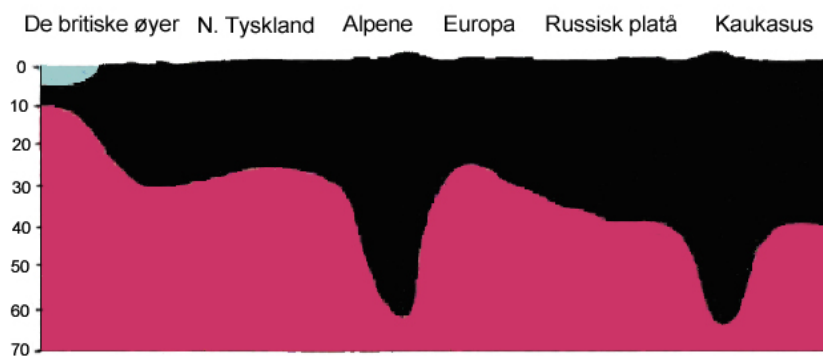
Figur 8: Schematisk tvärsnitt. Bergen har djupa pluggliknande rötter inbäddade i jorden. ( Anatomy of the Earth [Jordens anatomi], Cailleux, s. 220)
