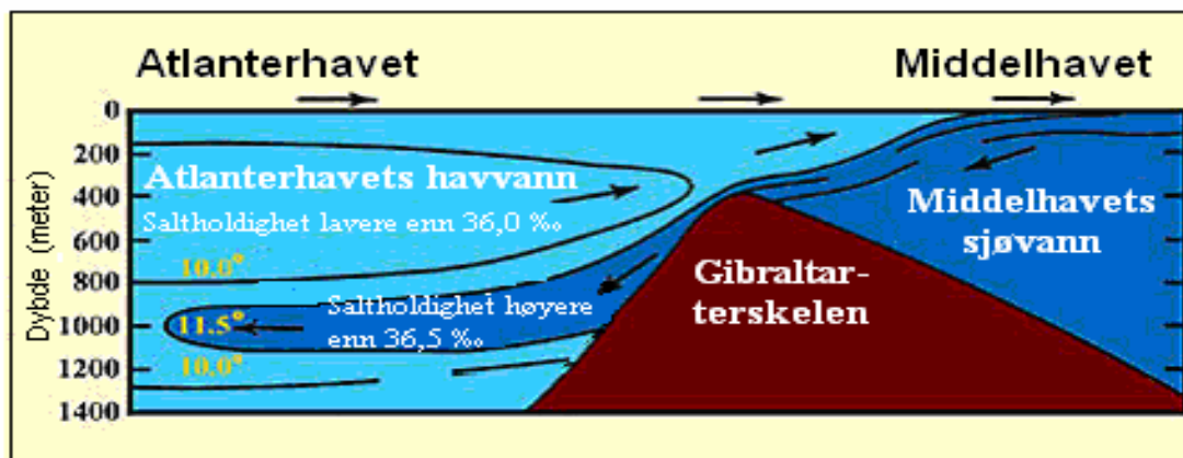
Figur 13: Medelhavets havsvatten flyter in i Atlanten över Gibraltarsträckan, och behåller sin egen temperatur, salthalt och mindre densitet egenskaper på grund av barriären som skiljer dem. Temperaturen anges i grader Celsius (°C). ( Marine Geology [Maringeologi], Kuenen, s. 43, med en liten förbättring)
