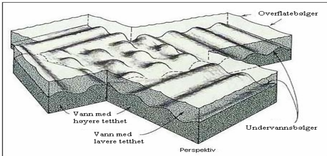
Figur 16: Undervattensvågorna på gränsen mellan två lager av vatten med olika densitet. Det nedre lagret har högre densitet, och det övre lagret har lägre densitet. ( Oceanography [Oceanografi], Gross, s. 204)
