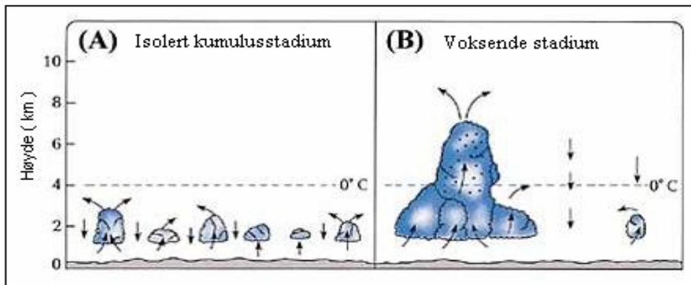
Figur 19: (A) Isolerade smådelar av moln (cumulusmoln). (B) När de små molnen samlas, ökar uppdrivningen i det större molnet, så att molnen staplas uppåt. Vattendroppar är indikerade med •. ( The Atmosphere [Atmosfären], Anthes m fl., s. 269)
