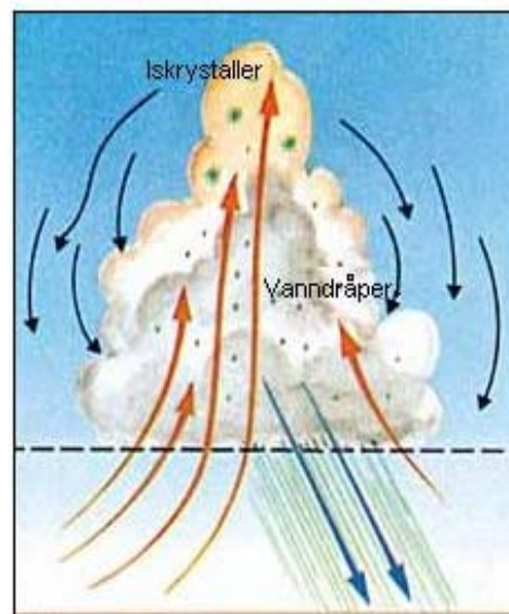
Figur 20: En cumulonimbusmoln (tordenmoln). Efter att molnet har staplats uppåt, kommer det regn ut ur den. ( Weather and Climate [Väder och klimat], Bodin, s. 123)
