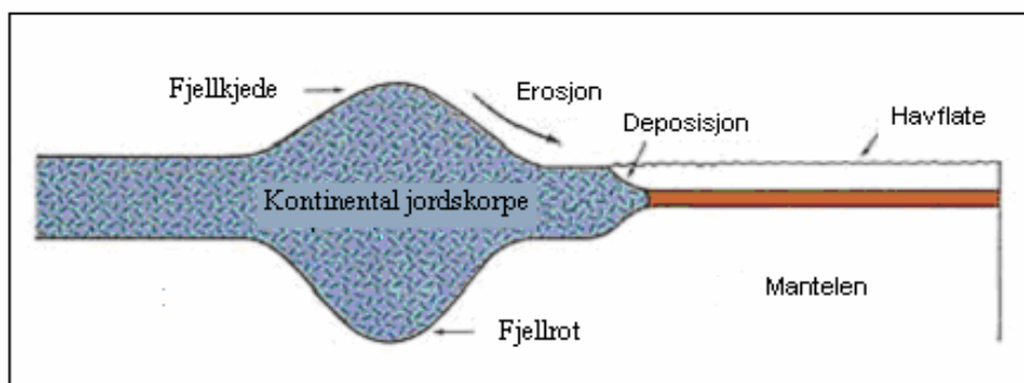
Figur 9: Denna illustration visar hur bergen på grund av de djupa rötterna, har pluggliknande form. ( Earth Science [Vetenskap om jorden], Tarbuck och Lutgens, s. 158)
