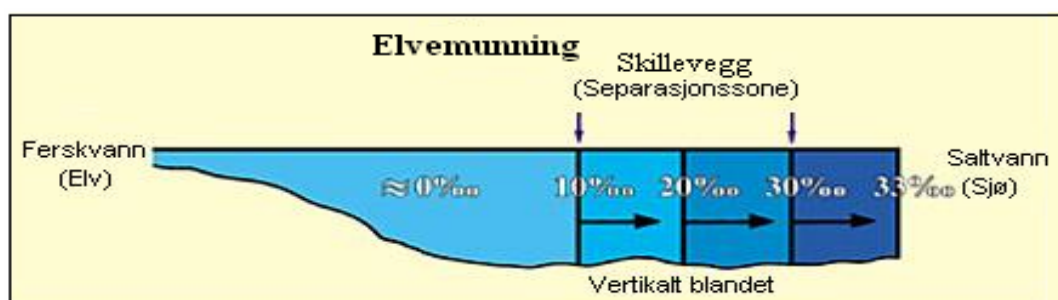
Figur 14: Längdsnitt som viser salthalten (i promille ‰) i en älvmyning. Här ser vi skiljeväggen (separationszonen) mellan färskvatten och saltvatten. ( Introductory Oceanography [Inledande oceanografi], Thurman, s. 301, med en liten förbättring)
