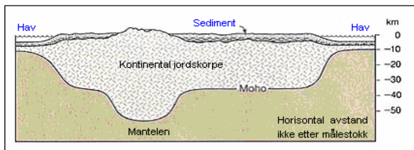
Figur 7: Bergen har djupa rötter under jordens yta. ( Earth [Jorden], Press och Siever, s. 413)
